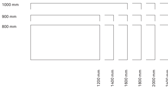
Arbeitstisch mit Raster-Höheneinstellung
